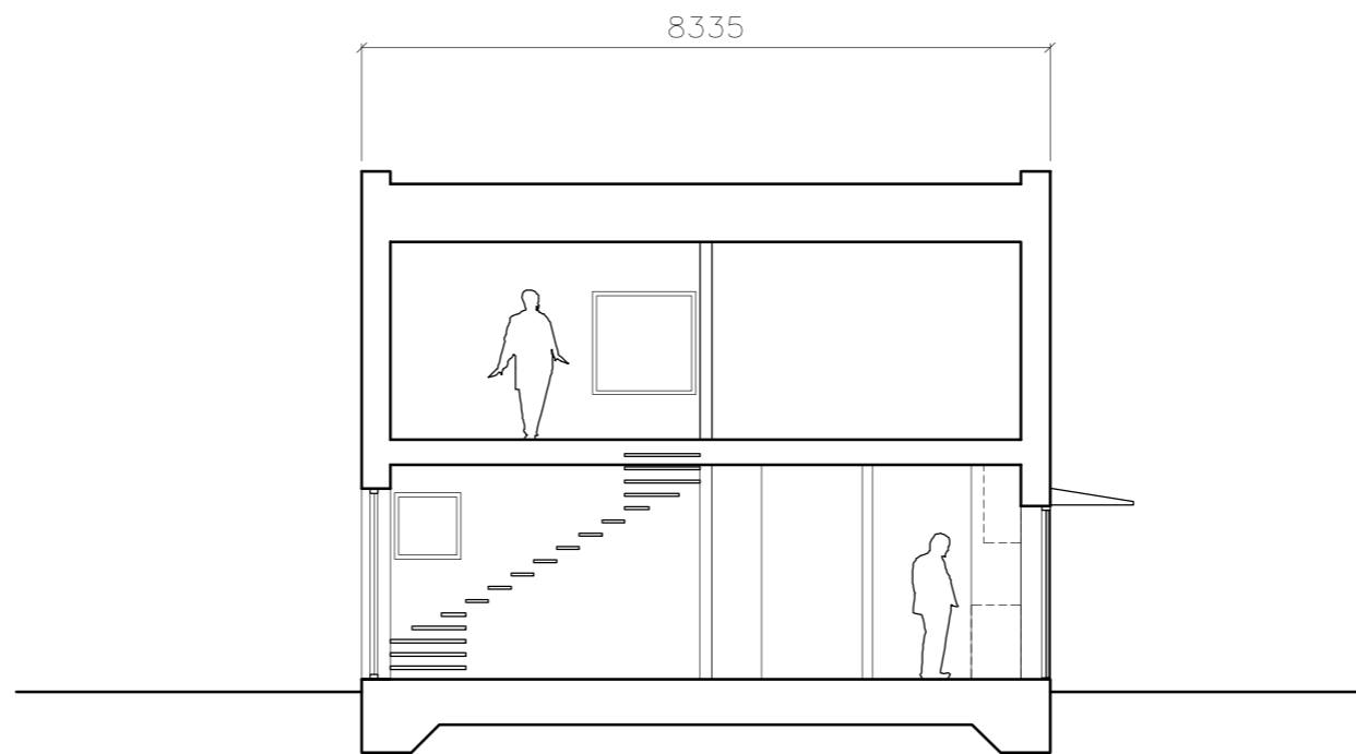
SEKTION A-A
