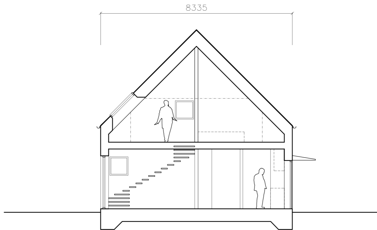
SEKTION A-A
