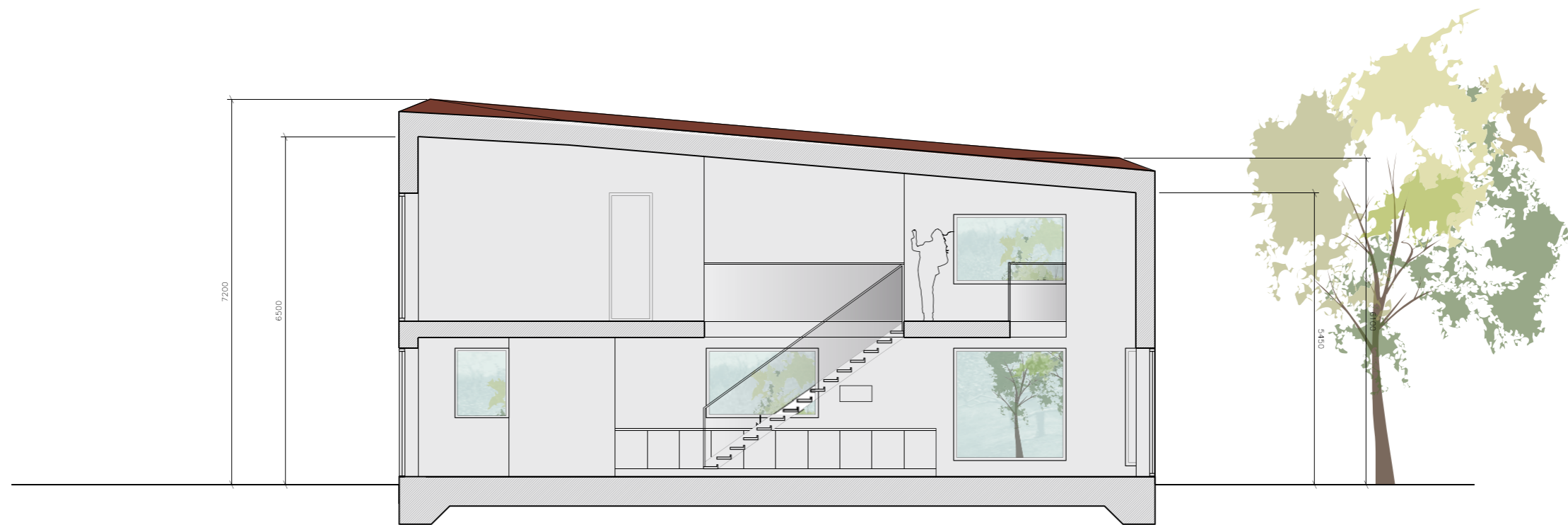
SEKTION A-A
